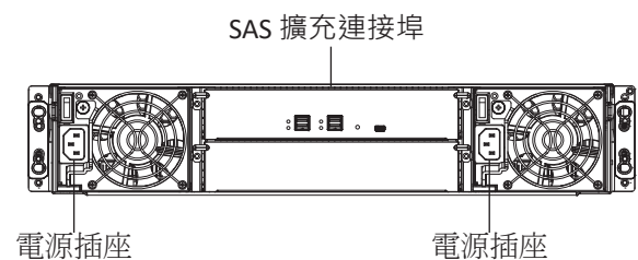
背板
