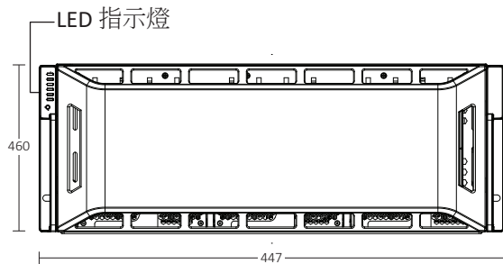
前面板 DS2460L-JB
